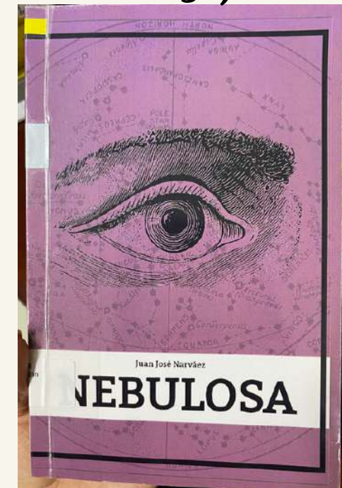
Nebulosa
